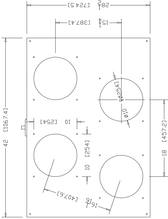
WSB-240 LID TOP VIEW
